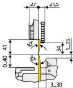
Altezza massima del componente presso la scanalatura preincisa
