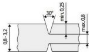
La scanalatura preincisa può essere interrotta da tacche fresate
